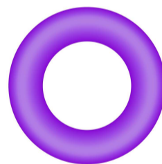
torus
